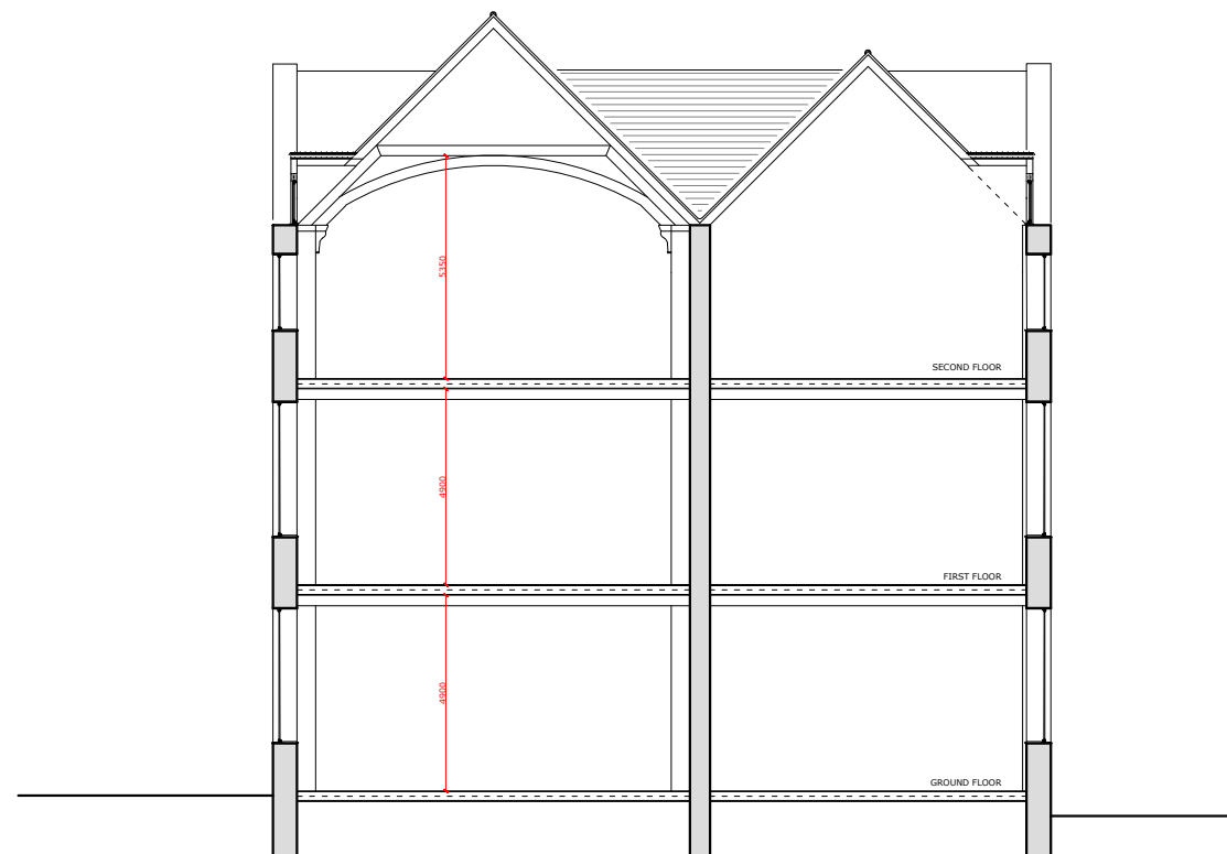
EXISTING SECTION SCALE: 1/200 @A3
